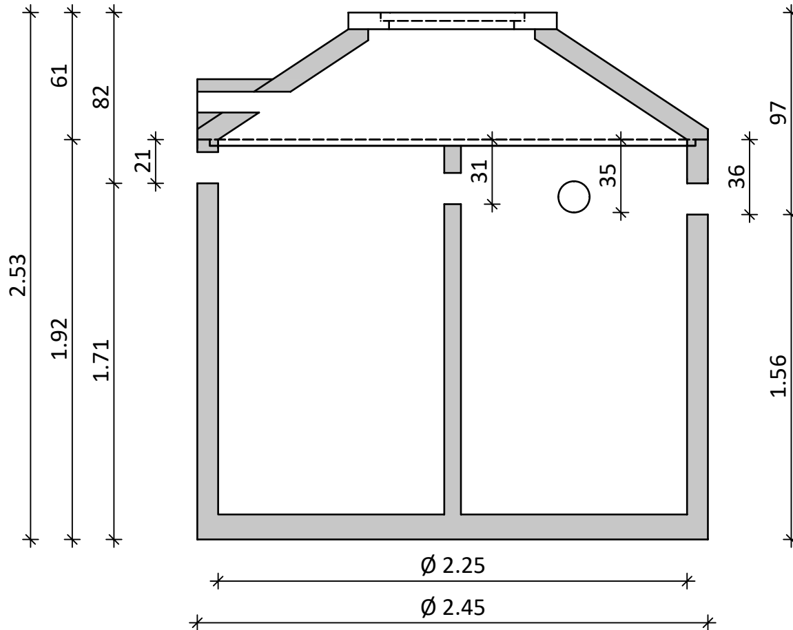
Konusabdeckung, Kl. A
